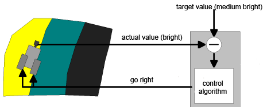
Boucle de régulation
